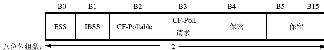
图4 能力信息固定字段
