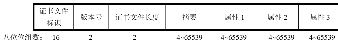
图16 证书颁发格式
