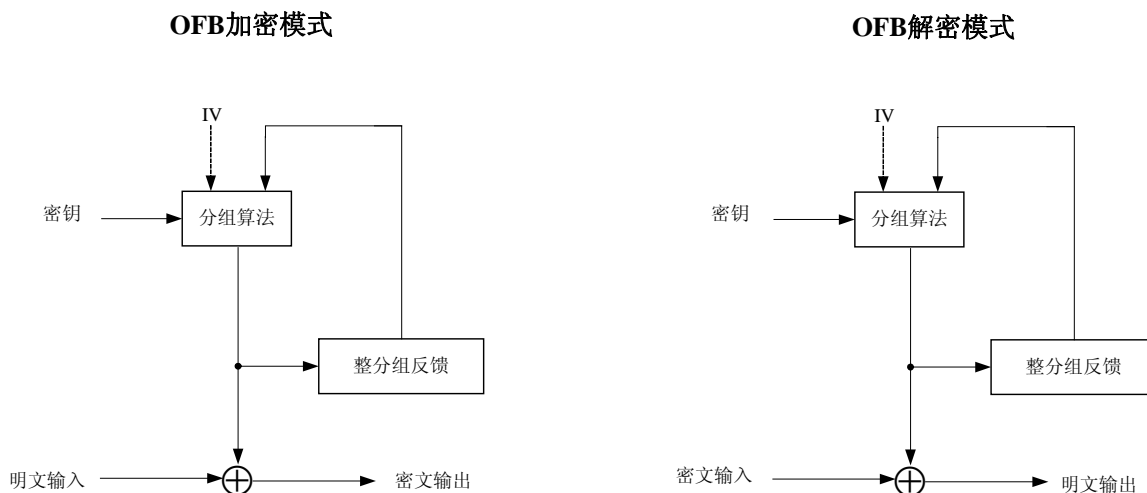
图49 工作模式
