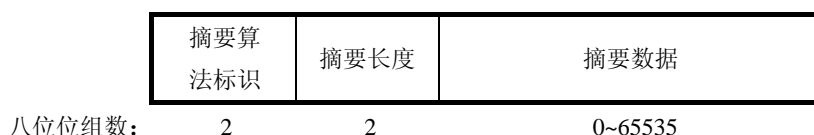
图17 摘要字段
