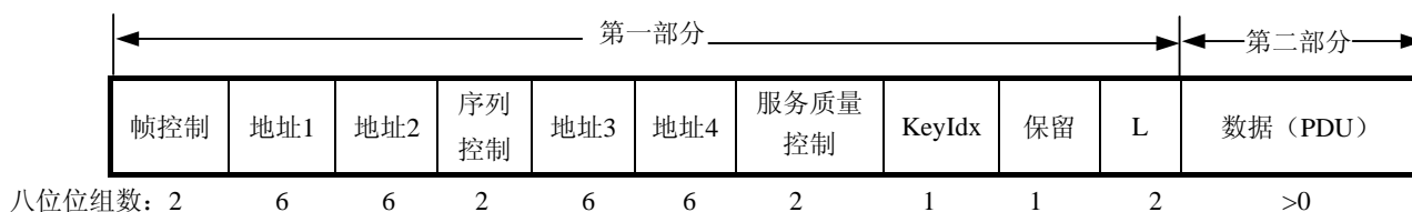
图51 完整性校验数据
