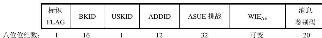
图38 单播密钥协商确认分组数据字段格式
