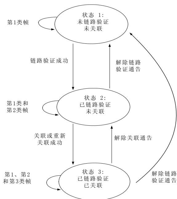
图1 状态转换图
